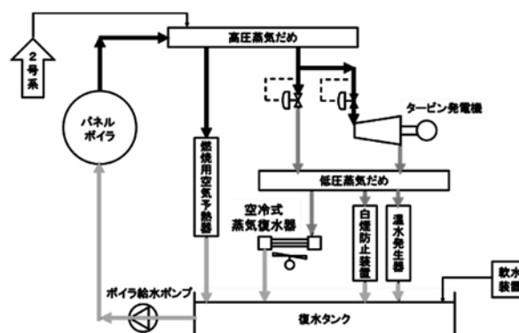
図 2 発電システム例
