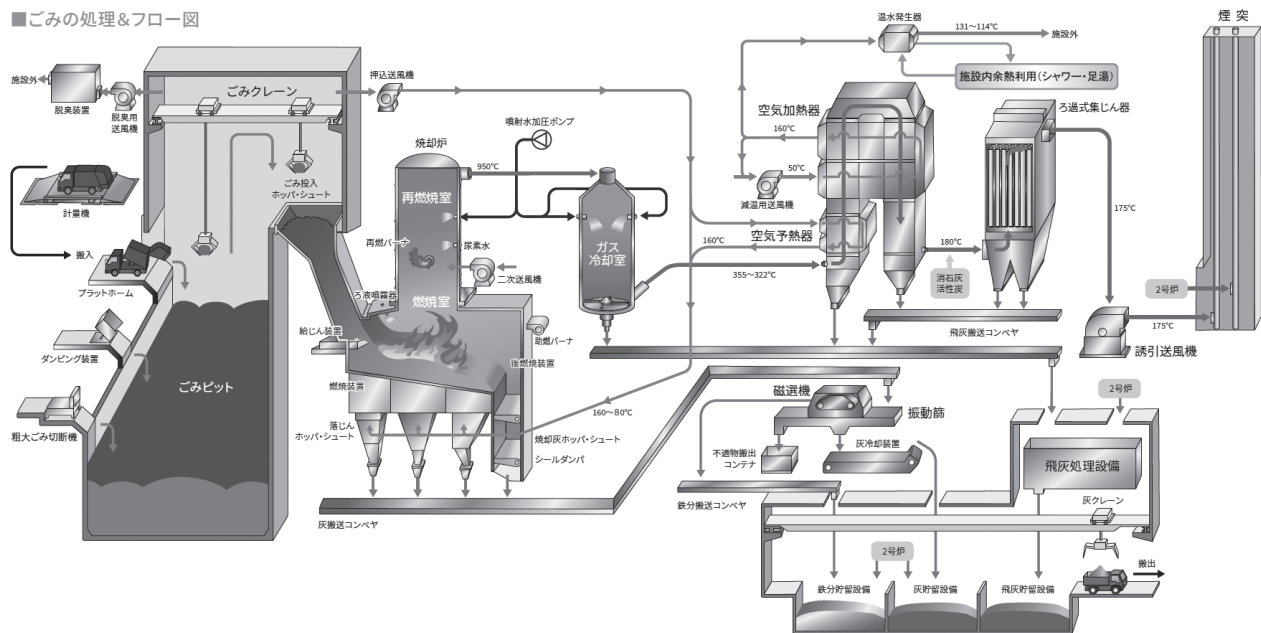
焼却施設フローシート
